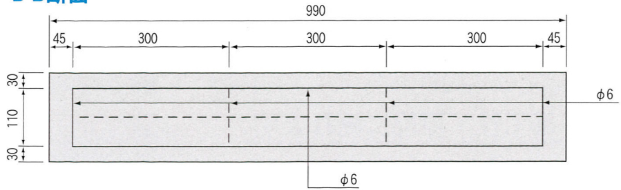
B-B断面
