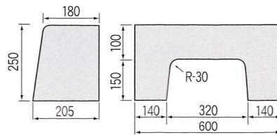
水抜 B W=48kg
