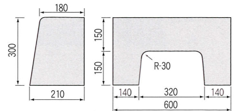
水抜 C W=57kg
